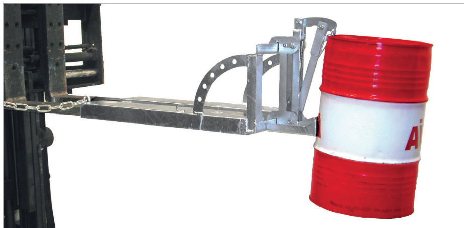
RS 60-I, inzetbaar voor vaten vanaf 500 mm hoogte met velsrand
